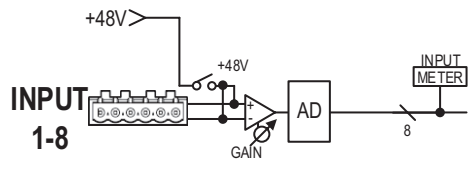
信号流
